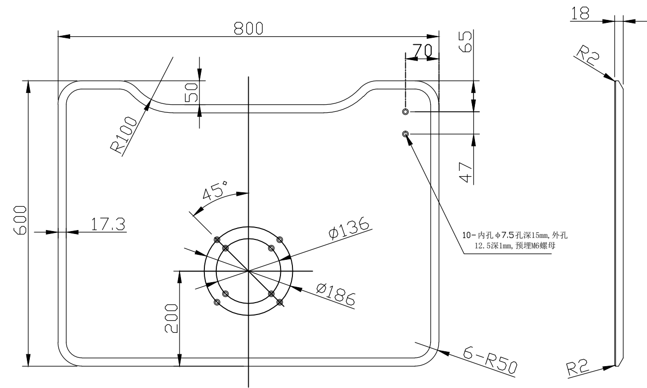
桌面800x600x18 双吸
